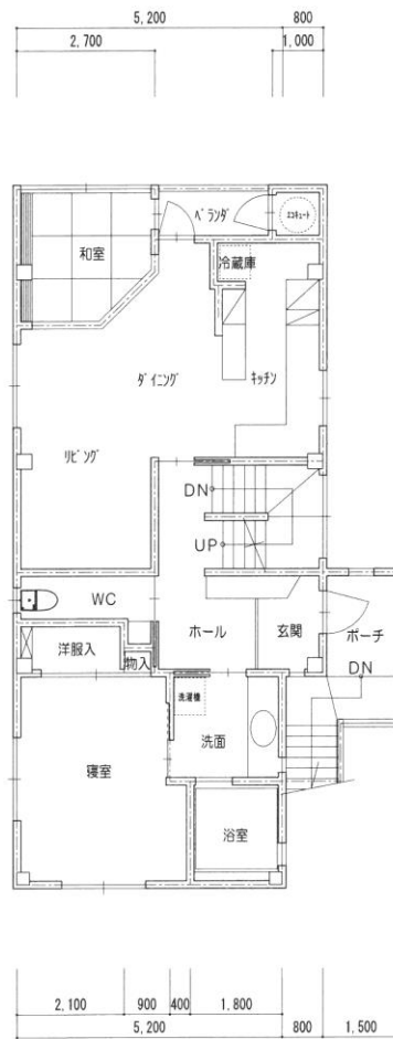
2階平面図 S=1/100
