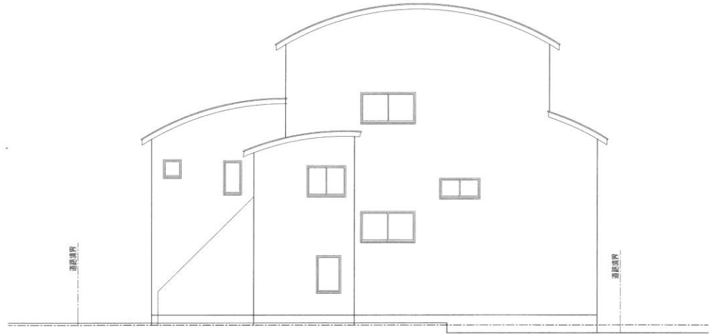
西侧立面图 S=1/100
